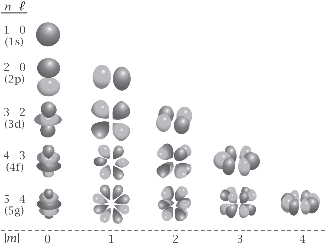
شكل ٨-٤: المدارات s، p، d، و f.
