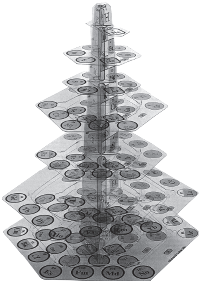
شكل ١٠-٢: شجرة دوفور الدورية.
