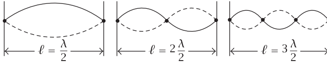
شكل ٨-٣: الشروط الحدية و بروز صفة الكمية.
