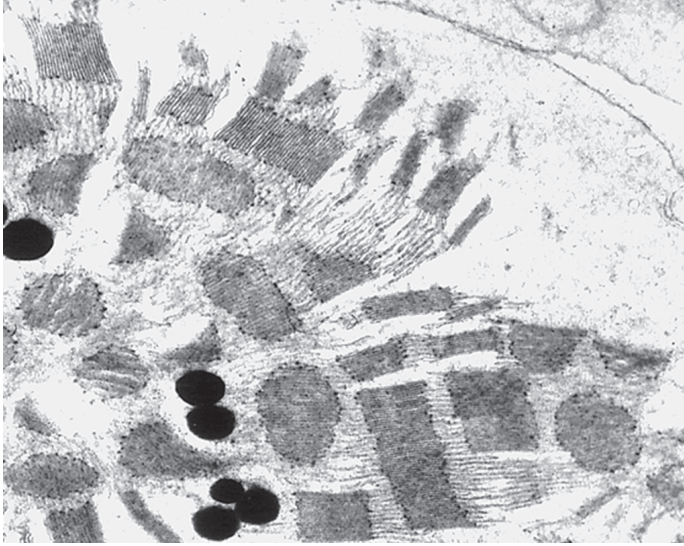
شكل ٤-٣: تلتقط النباتات أشعة الشمس، وتحولها إلى طاقة كيميائية في البلاستيدات الخضراء، التي تمتلئ بتلك «الملاءات» أو اللويحات المكسدة التي تسمى «الأغشية الثايلاكويدية».
