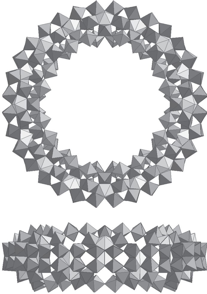
شكل ١-١٠: «عجلة كبيرة» من الجزيئات صنعتها مجموعة أليم مولر في ألمانيا (من منظور علوي وجانبي). يتكون كل هرم منها من مجموعة من ذرات الموليبدنوم والأكسجين.
