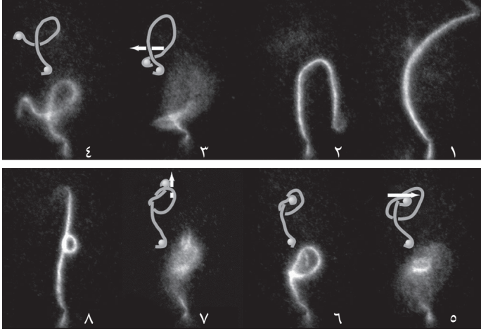
شكل ٥-٥: استُخدم الملقط البصري لربط هذه العقدة في خيط من الأكتين. عملت الخرزتان المجهريتان المتصلقتان بكلتا نهايتي الخيط «كمقبضين»، وقد تم إظهار الأكتين للعيان تحت المجهر بتسليط الضوء الساطع عليه لجعله متألقاً.
