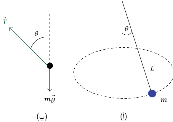
شكل ١١-٣: رسم توضيحي (أ) ومخطط الجسم الحر (ب) للمثال ١٢-٣.
