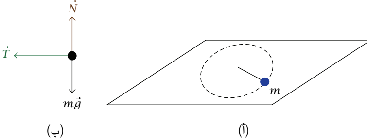
شكل ١٠-٣: رسم توضيحي (أ) ومخطط الجسم الحر (ب) للمثال ١١-٣.
