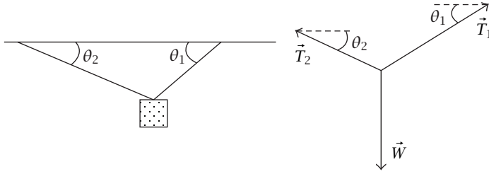
شكل ٦-٢: رسم توضيحي ومخطط الجسم الحر للمثال ٢-٤.
