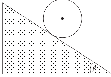
شكل ٨-٢٤: كرة مصمتة تتدحرج بدون انزلاق على منحدر لأسفل.
