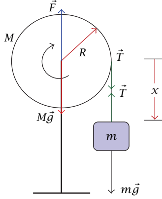
شكل ٨-١١: القوى المؤثرة على القالب والحداقة في مثال ٨-٣.
