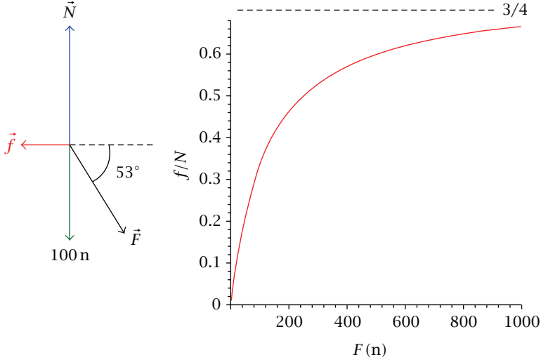
شكل ٢-٢١: منحني بياني لـ f/N مقابل F لمثال ٢-١٢ (ج).
