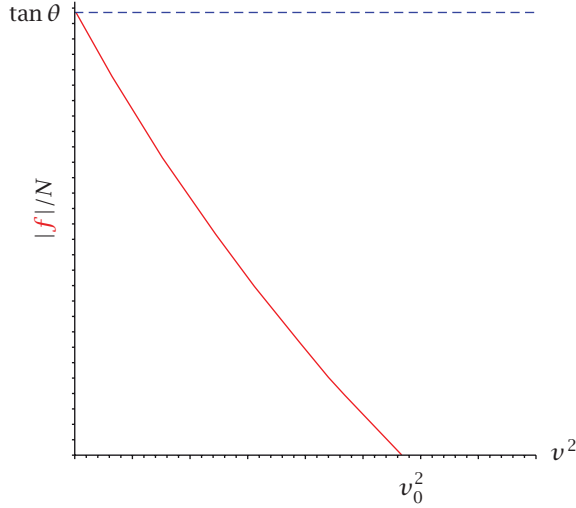
شكل ٣-١٤: الرسم البياني لنفس النسبة عندما يكون مقدار السرعة أقل من v_0 .
