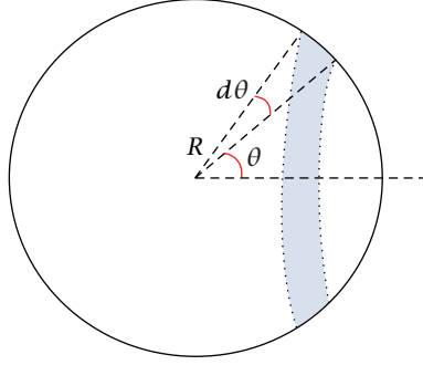
شكل ٨-٢٣: قسمنا الكرة الجوفاء بمستويات عمودية على محور.
