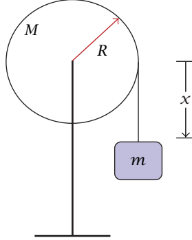
شكل ٨-٢٩: عجلة حدافة كتلتها M ، وثقل كتلته m مع إزاحة مسافة x في الاتجاه الرأسي.
