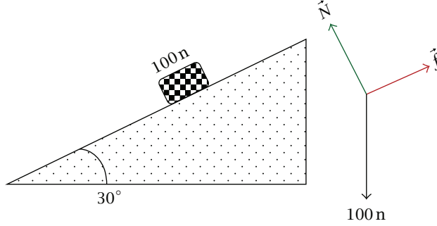
شكل ١٦-٢: الرسم التوضيحي ومخطط الجسم الحر لمثال ١٠-٢.
