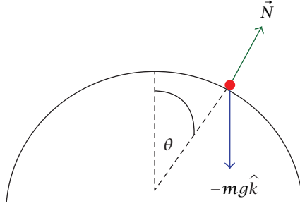
شكل ٥-٦: مخطط بيان القوة لجُسيم ينزلق على سطح نصف كروي في المثال ٥-٢.
