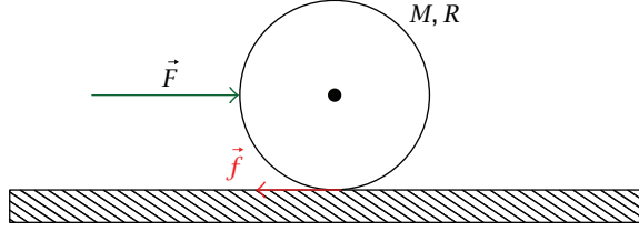
شكل ٨-٢٦: ضُربت كرة بلياردو بقوة دفعية كبيرة بما يكفي لأن تبدأ الكرة الدحرجة بانزلاق في المثال ٨-٨.
