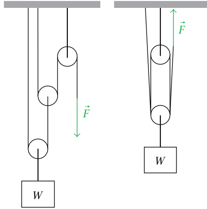
شكل ٢-١٢: كلٌّ من هذين الترتيبين للبكرات يوفر أربعة أضعاف الفائدة الميكانيكية.
