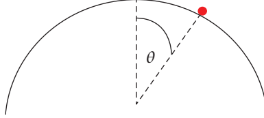
شكل ٥-٥: جُسيم يبدأ من السكون عند قمة نصف كرة وأعطى دفعة متناهية في الصغر في مثال ٥-٢.
