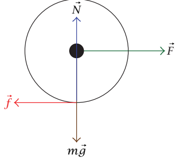
شكل ٨-٢٢: القوى المؤثرة على إحدى عجلات العربة. \vec{F}' هي القوة الأفقية التي يبذلها المحور، و \vec{N} هي مجموع القوى الرأسية التي تبذلها الأرض على المحور.
