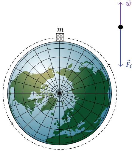
شكل ٩-١: مسقط عمودي لصورة الكرة الأرضية كما يُرى من فوق القطب الشمالي مباشرة. الكتلة m تدور مع سطح الأرض. نرغب في تحديد تأثير دوران الأرض على الوزن w .
