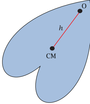
شكل ٨-١٦: جسم اختياري الشكل وحر لأن يتذبذب حول نقطة O تحت تأثير الجاذبية. انظر المثال ٨-٥.
